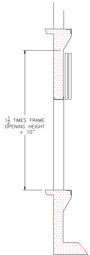
ELEVATION
